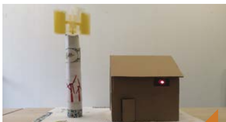
Fabrication d'une mini éolienne
